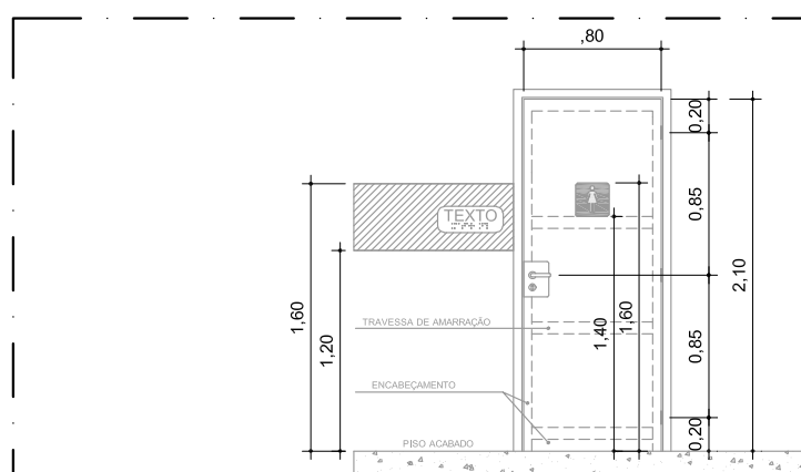
DET. GENÉRICO - SINALIZAÇÃO TÁTIL E VISUAL ESC.: 1:50
